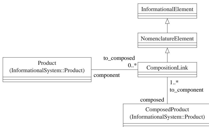
FIG. 9.8 – Extrait du métamodèle du sous-système informationnel
