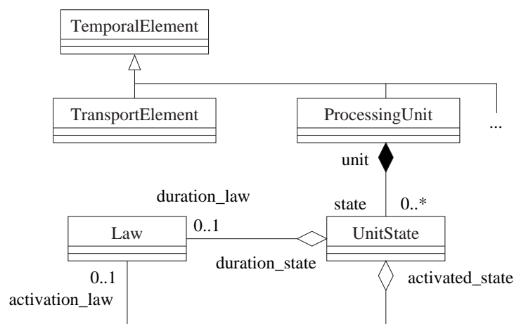
FIG. 9.7 – Extrait du métamodèle du sous-système opérationnel
