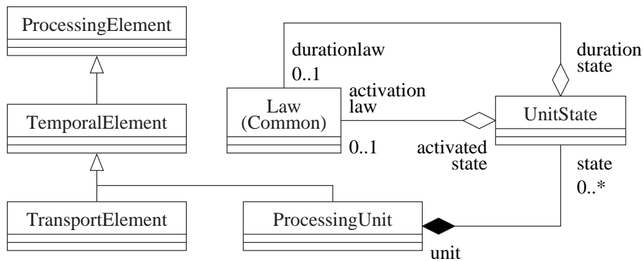
FIG. A.8 – Simulation::PhysicalFlow : Eléments avec traitement temporisé
