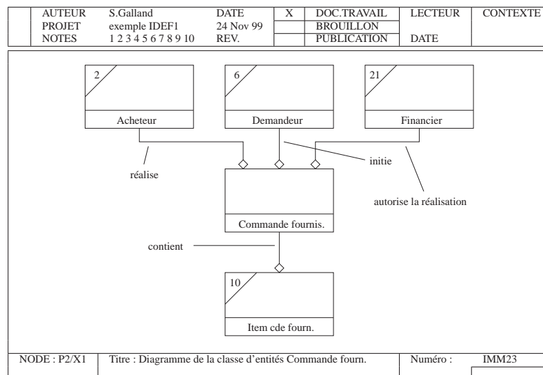
FIG. 4.2 – IDEF1 – Diagramme de classes d'entités
