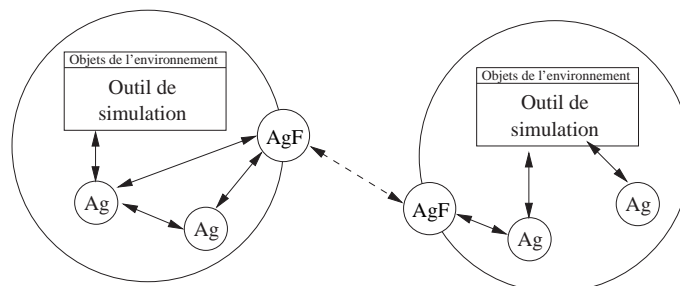
FIG. 11.1 – Architecture du SMA de simulation
