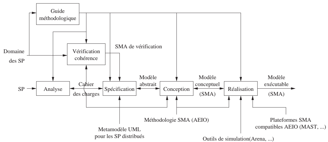
FIG. 8.3 – Cycle de vie – Démarche en cascade durant une itération
