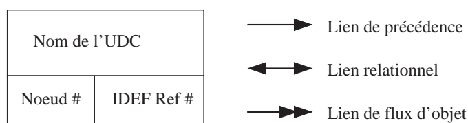
FIG. 4.3 – IDEF3 - Constructions de base
