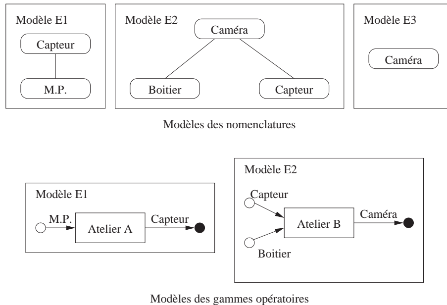
FIG. 9.4 – Exemple de modèles du sous-système informationnel
