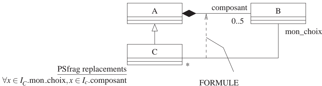
FIG. 9.9 – Extrait d'un métamodèle pour la vérification locale
