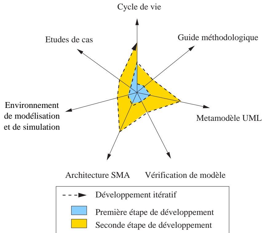
FIG. 2.2 – Développement itératif de M CA M SA -S
