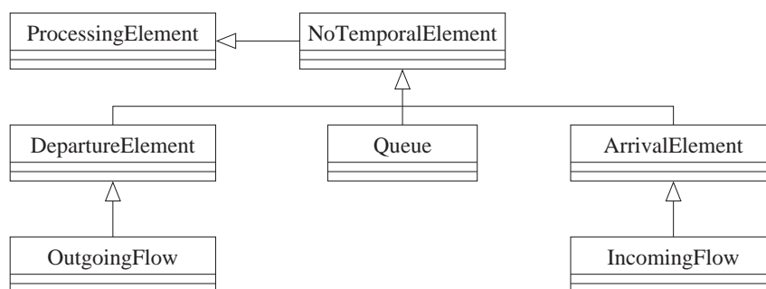
FIG. A.6 – Simulation::PhysicalFlow : Éléments avec traitement immédiat
