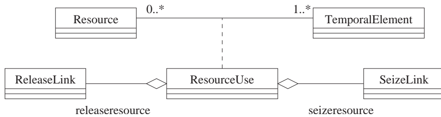
FIG. A.4 – Simulation::PhysicalFlow : Allocation et libération de ressources
