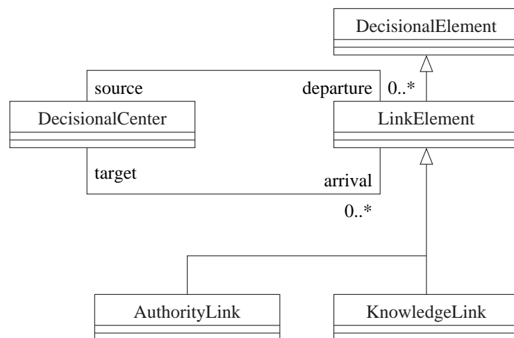
FIG. A.26 – Simulation::DecisionalProcess::Organization : Liens décisionnels
