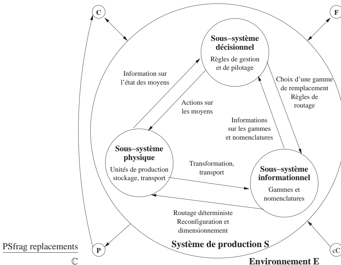
FIG. 5.2 – Système de production S plongé dans son environnement E
