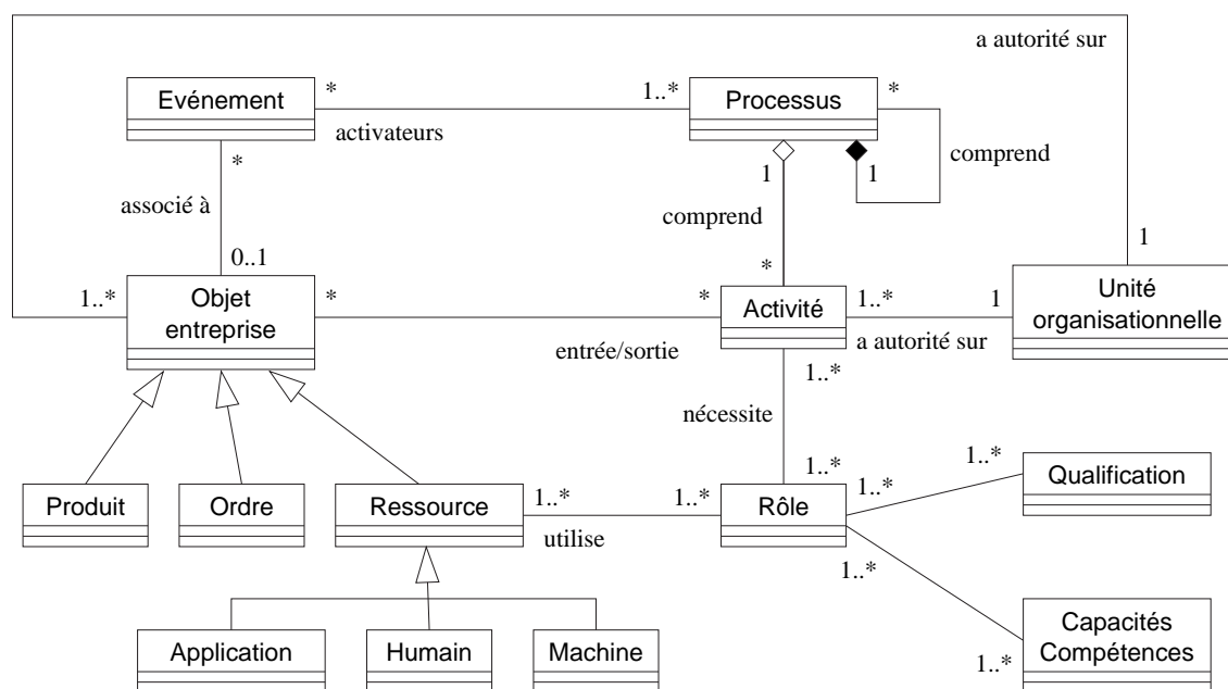
FIG. 4.6 – Éléments principaux de modélisation d'UEML [ VERNADAT, 2001 ]
