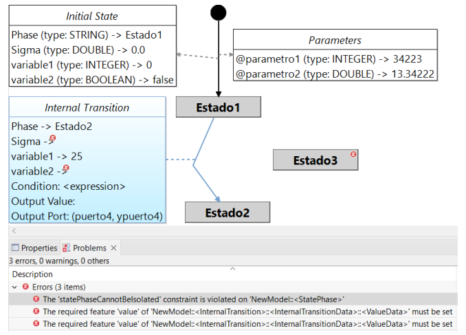
Fig. 5. Validación de instancia. La fase Estado3 viola la restricción de no existencia de fases aisladas; mientras que la transición interna entre Estado1 y Estado2 tiene dos campos obligatorios sin configurar.
