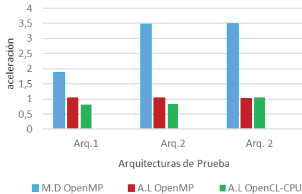
Fig. 11 Aceleración obtenida en las arquitecturas de prueba con 4350 trazas.
