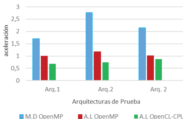
Fig. 10 Aceleración obtenida en las arquitecturas de prueba con 2350 trazas.
